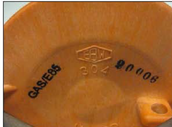
EBW 30420006 Vapor Dust Cap (Gas/E85)
